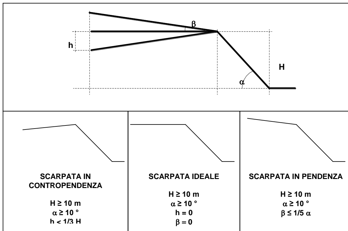
Figura 1 – Schematizzazione delle tipologie di scarpata
